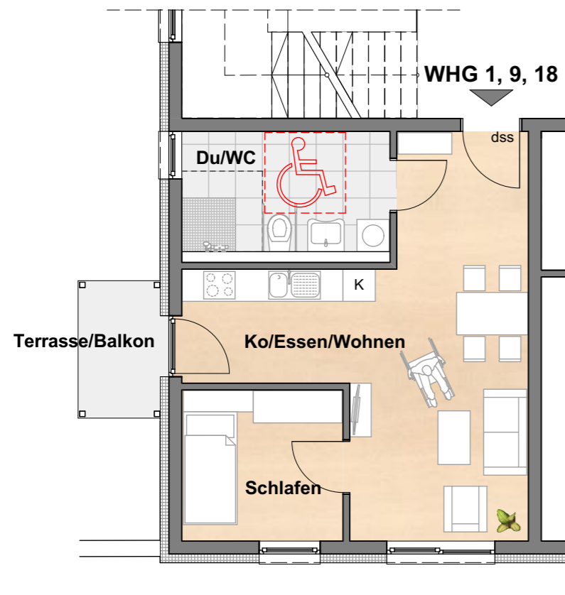
GRUNDRISS im MA&STAB 1 : 100
